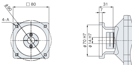
図6 0.4kW T2, T4
