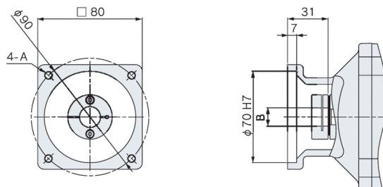
図4 0.2kW T2, T4
