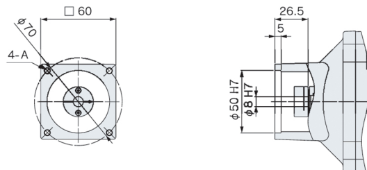
図2 0.1kW T2, T4
